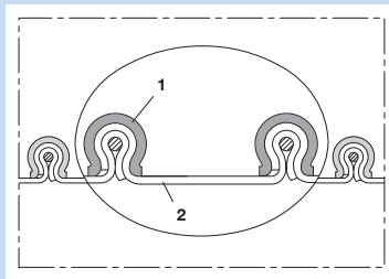
Hochtemperaturschlauch, Klemmprofilschlauch, (bis +450°C)
