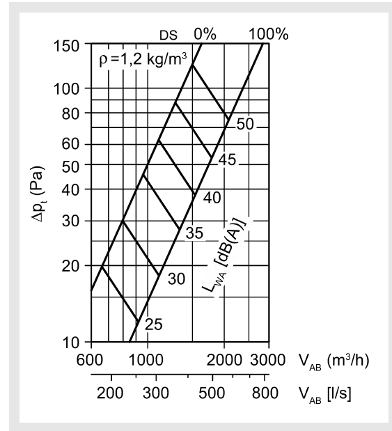
DQJ-...-SR-A-600/625-...
