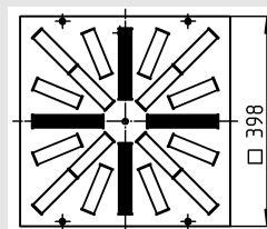
DQJ-Q/S-SQ-Z-400-...
