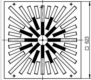
DQJ-Q/S-SQ-Z-625-...
