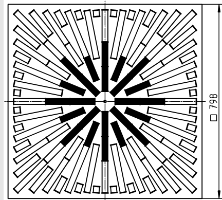
DQJ-Q-SQ-Z-800-...
