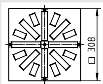
DQJ-Q/S-SR-Z-310-...-PS-...
