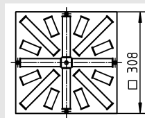
DQJ-Q/S-SQ-Z 310-...-PS-...
