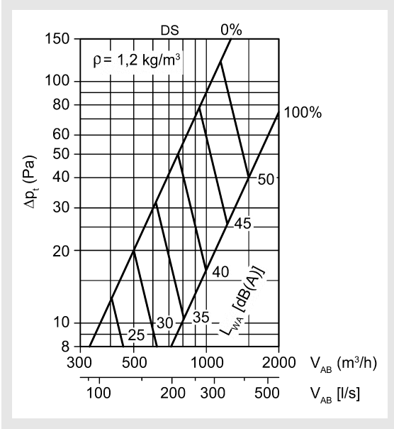
DQJ-...-SQ-A-500-...
