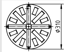
DQJ-R-SR-Z-310-...-PS-...
