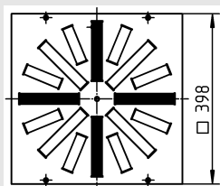
DQJ-Q/S-SR-Z-400-...-PS-...
