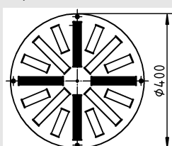
DQJ-R-SR-Z-400-...-PS-...
