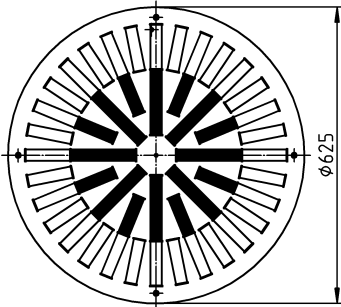
DQJ-R-SR-Z-625-...
